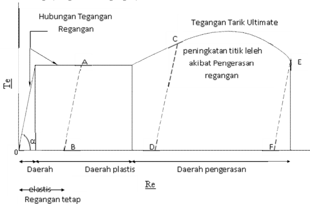
Gambar 2. Bentuk kurva ideal hubungan tegangan–regangan akibat adanya regangan yang melebihi pada daerah elastis. (Charles G Salmon (1991))
