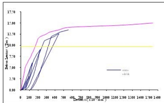
Gambar 12. Kurva Hubungan Beban Lentur Dan Defleksi Balok Dengan Penulangan Baja Mutu 400 Mpa Untuk Pengujian Rencana, Monotonik Dan Statis Siklik
