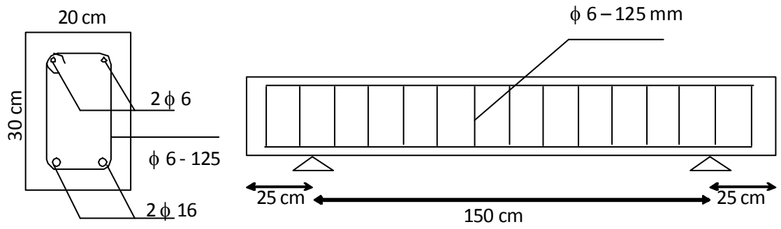
Gambar 3. Detail Pengujian Balok
