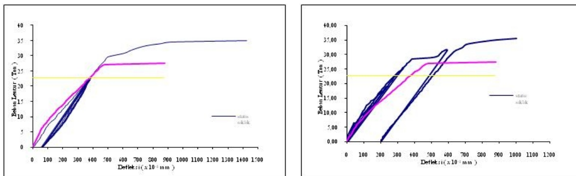
Gambar 11. Kurva Hubungan Beban Lentur Dan Defleksi Balok Dengan Penulangan Baja Mutu 240 Mpa Untuk Pengujian Rencana, Monotonik Dan Statis Siklik
