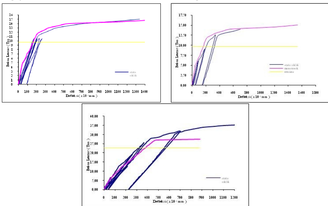
Gambar 11. Kurva Hubungan Beban Lentur Dan Defleksi Balok Dengan Penulangan Baja Mutu 240 Mpa Untuk Pengujian Rencana, Monotonik Dan Statis Siklik
