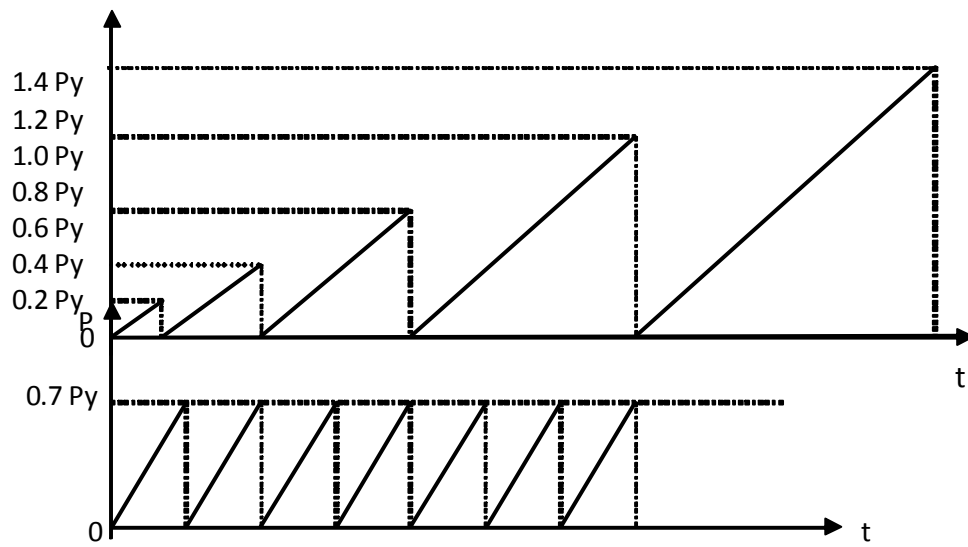
Gambar 4. Pola pembebanan pengujian statis siklik
