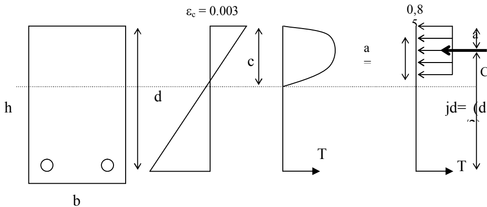
Gambar 1. Distribusi Tegangan Dan Regangan Pada Balok.
