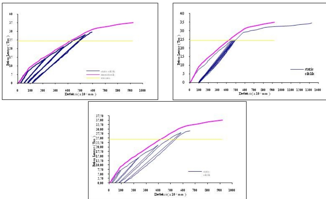
Gambar 13. Kurva Hubungan Beban Lentur Dan Defleksi Balok Dengan Penulangan Baja Mutu 500 Mpa Untuk Pengujian Rencana, Monotonik Dan Statis Siklik.
