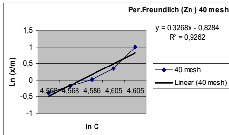
Gambar 6. Kurva isotherm Freundlich untuk adsorpsi Zn dengan zeolit
