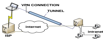
Gambar 2: Koneksi VPN
