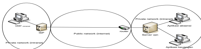
Gambar 3 : Simulasi VPN
