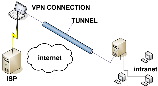
Gambar 4: Koneksi VPN
