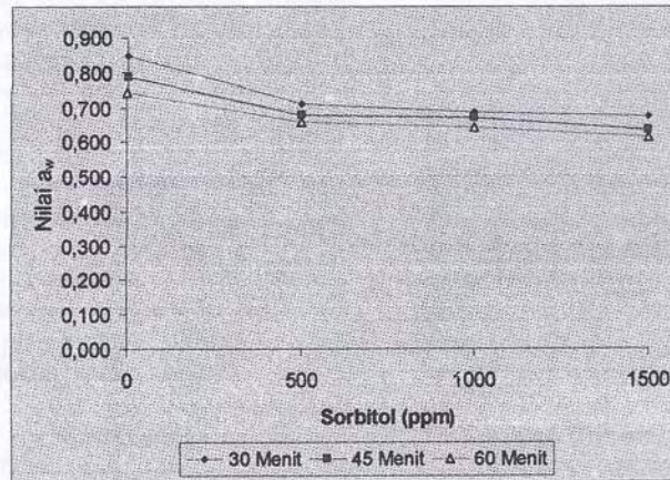
Gambar 2. Hubungan antara penambahan sorbitol dan lama pengovenan terhadap a_w getuk pisang oven
