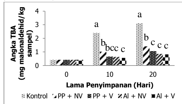
Gambar 4. Pengaruh Jenis Kemasan Terhadap Angka TBA Bumbu Ayam Taliwang Khas Lombok Selama Penyimpanan: Keterangan: Huruf yang sama pada grafik menyatakan hasil yang tidak berbeda nyata.
